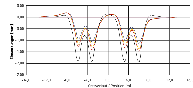
Beispiel Einsenkung
