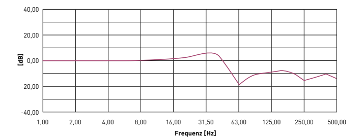
Beispiel Einfügungsdämmmaß
